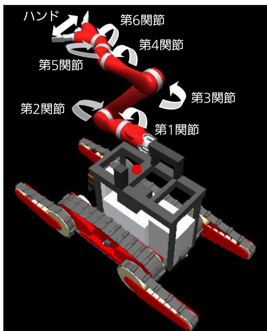
図 1.2: アーム操作方法
