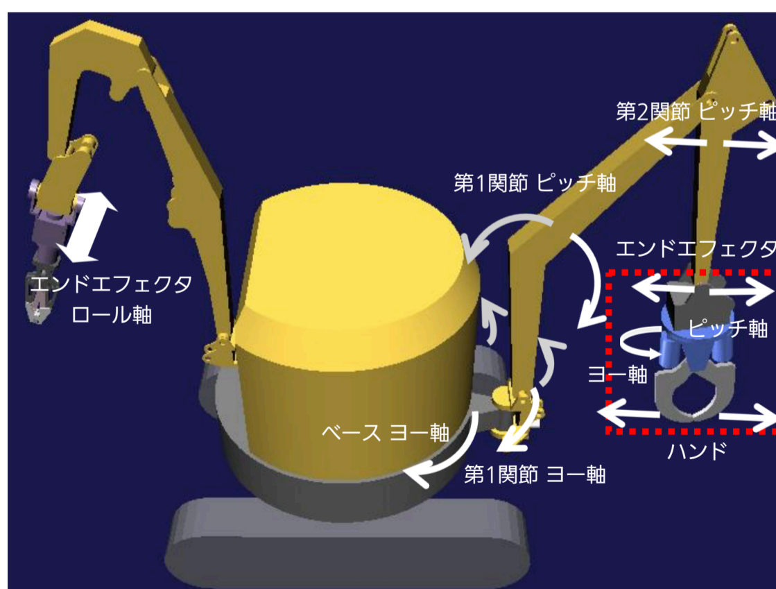
図 3.1: 双腕建機モデル操作方法
